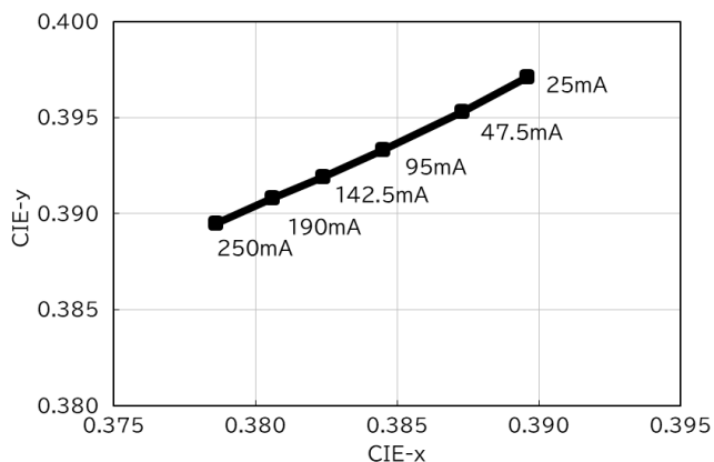
●順方向電流—色度特性 [Ta=25℃]
