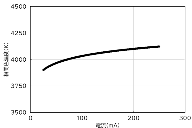
●順方向電流—色温度特性〔 T_a = 25^\circ\text{C} 〕
