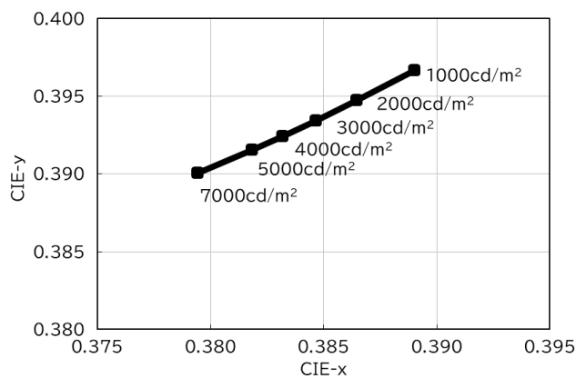
●輝度—色度特性 [Ta=25℃]
