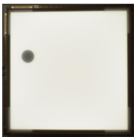
<図 5.3.1> 発光面に生じたダークスポットの例(ダークスポットの直径は約 8 mm)
