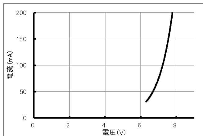
●順方向電流—電圧特性〔 T_a=25^\circ\text{C} 〕
