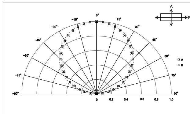
●配光分布〔順方向電流 I_f=95\text{mA} T_a=25^\circ\text{C} 〕
