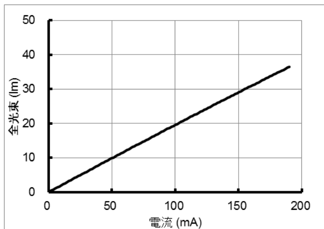
● 順方向電流—全光束特性 [Ta=25°C]
