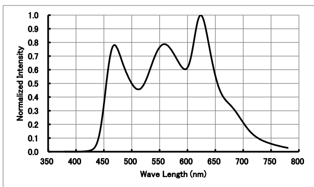
●分光分布〔順方向電流 I_f=95\text{mA} T_a=25^\circ\text{C} 〕
