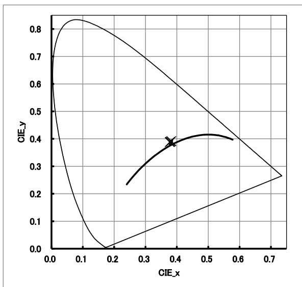
●色度図〔順方向電流 I_f=95\text{mA} T_a=25^\circ\text{C} 〕
