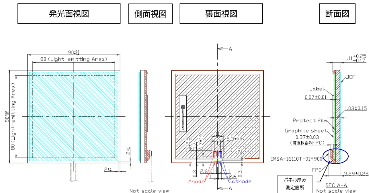
(図面 4) KN-P-P4-BK-40-U/FS (コネクタ実装 FPC タイプ)
