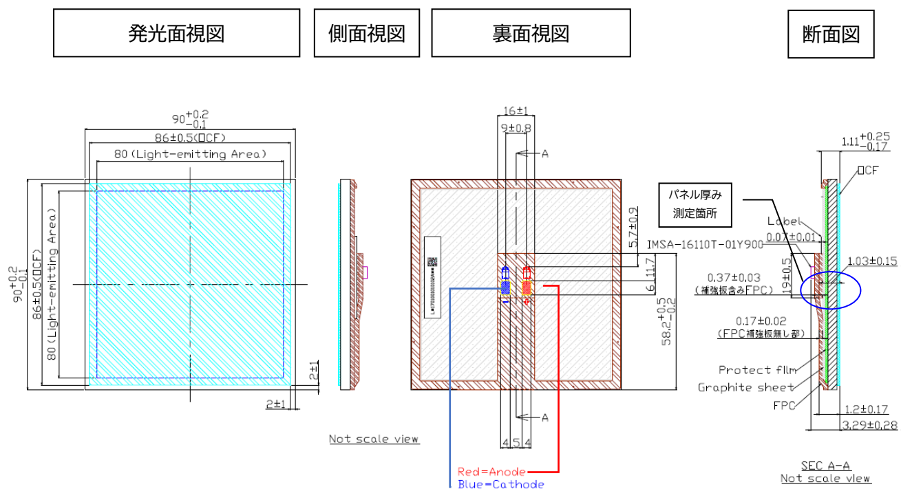
(図面 3) KN-P-P4-BK-40-U/FC (コネクタ実装 FPC タイプ)
