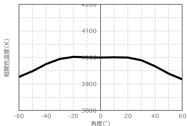
●角度依存性(色温度)
