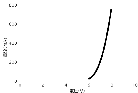
●順方向電流—電圧特性〔 T_a = 25^\circ\text{C} 〕
