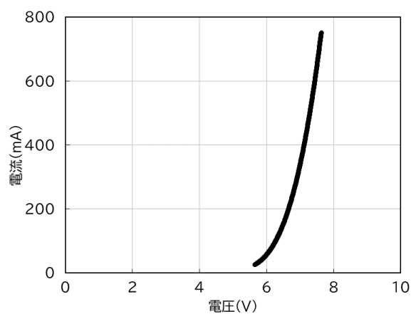
●順方向電流—電圧特性〔 T_a = 25^\circ\text{C} 〕
