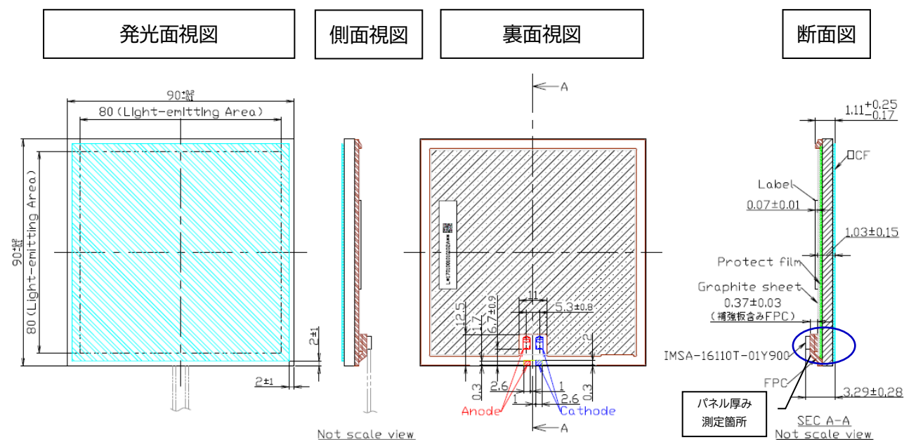
(図面 4) KN-P-HC-BK-30-U/FS (コネクタ実装 FPC タイプ)
