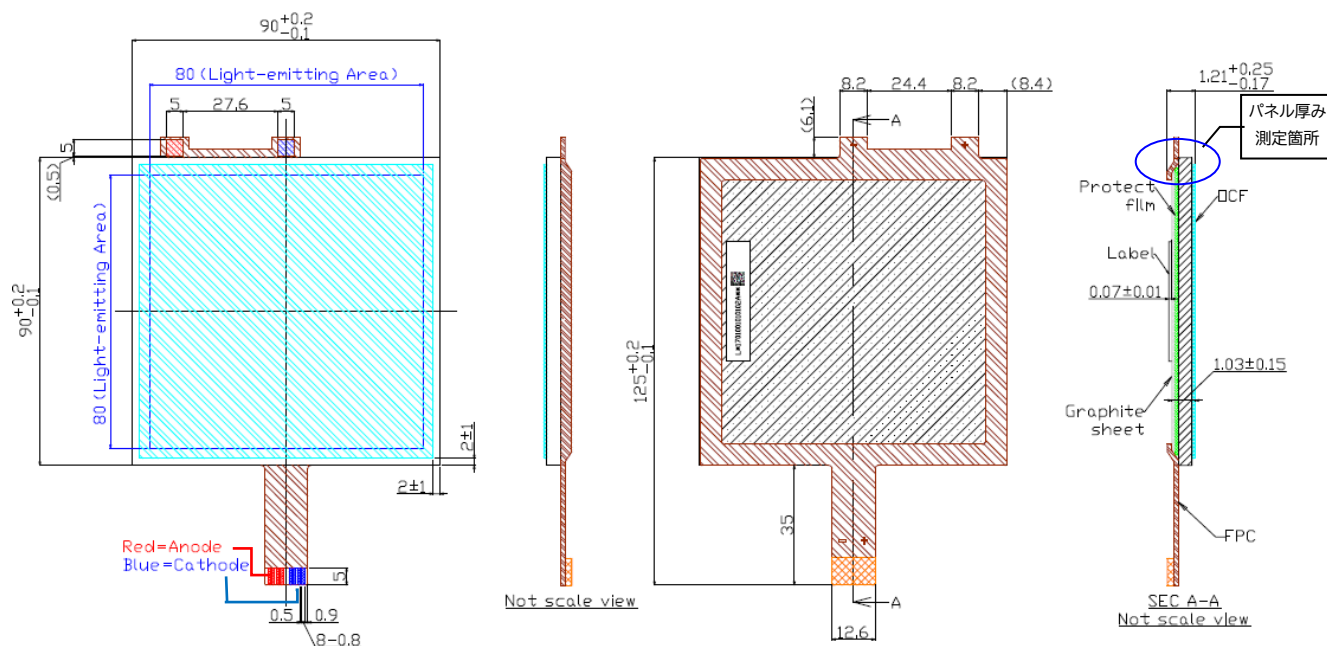
発光面視図
