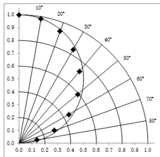
●配光分布〔順方向電流 I_f = 250\text{mA} T_a = 25^\circ\text{C} 〕
