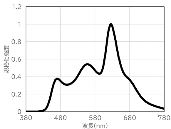
●分光分布〔順方向電流 I_f = 250\text{mA} T_a = 25^\circ\text{C} 〕
