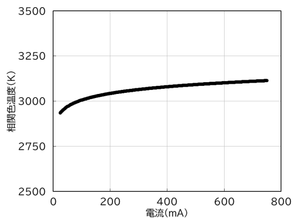
●順方向電流—色温度特性〔 T_a = 25^\circ\text{C} 〕
