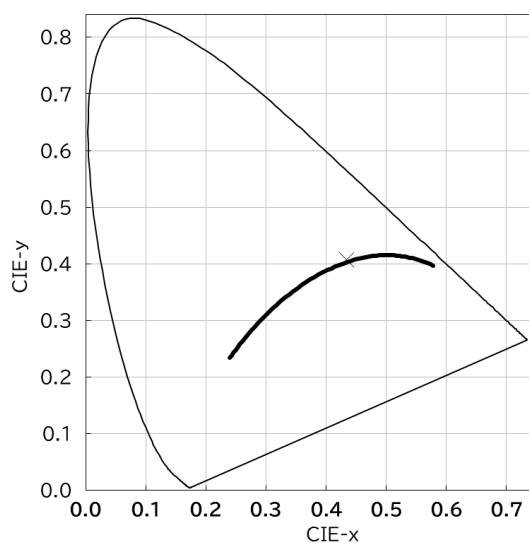
●色度図〔順方向電流 I_f = 250\text{mA} T_a = 25^\circ\text{C} 〕
