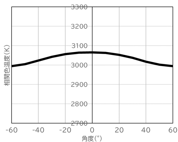
●角度依存性(色温度)
