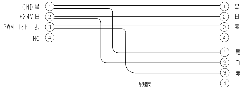
配線図
