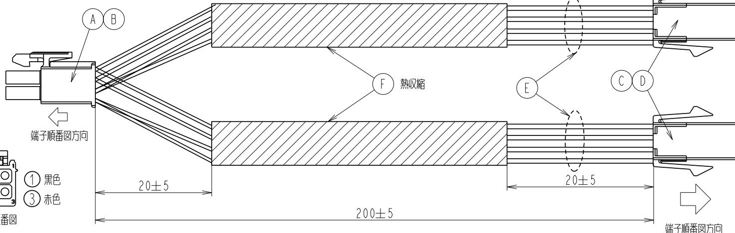
端子順番図方向
