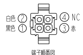
端子順番図
