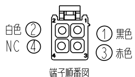
端子順番図
