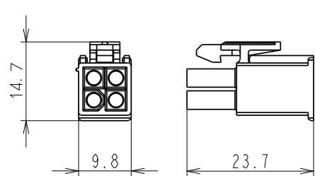
プラスチックケース外形寸法図
