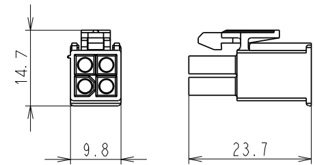
プラスチックケース外形寸法図
