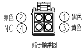
端子順番図
