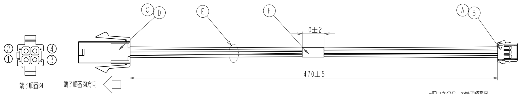
上記コネクタの端子順番図
