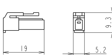
プラスチックケース外形寸法図 SLP-01V
