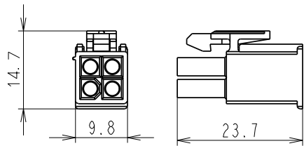
プラスチックケース外形寸法図 172167-1
