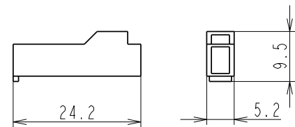
プラスチックケース外形寸法図 SLR-01VF
